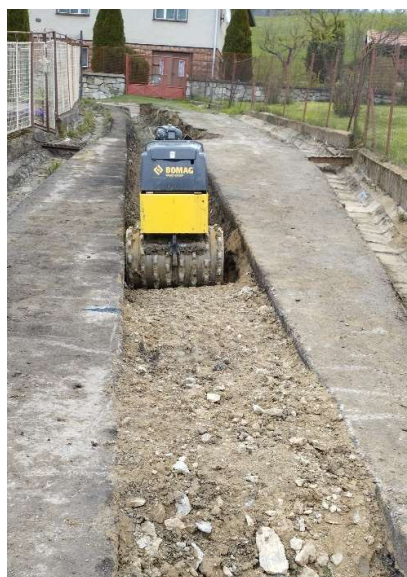
Obr. 2: Vibračné zhutňovanie zemin - spätný zásyp v obci Žaškov (SS.01)
